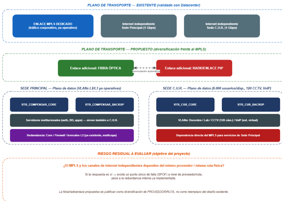
Figura N7 Escenario real validado (MPLS + redundancia existente) y propuesta de diversificación.
